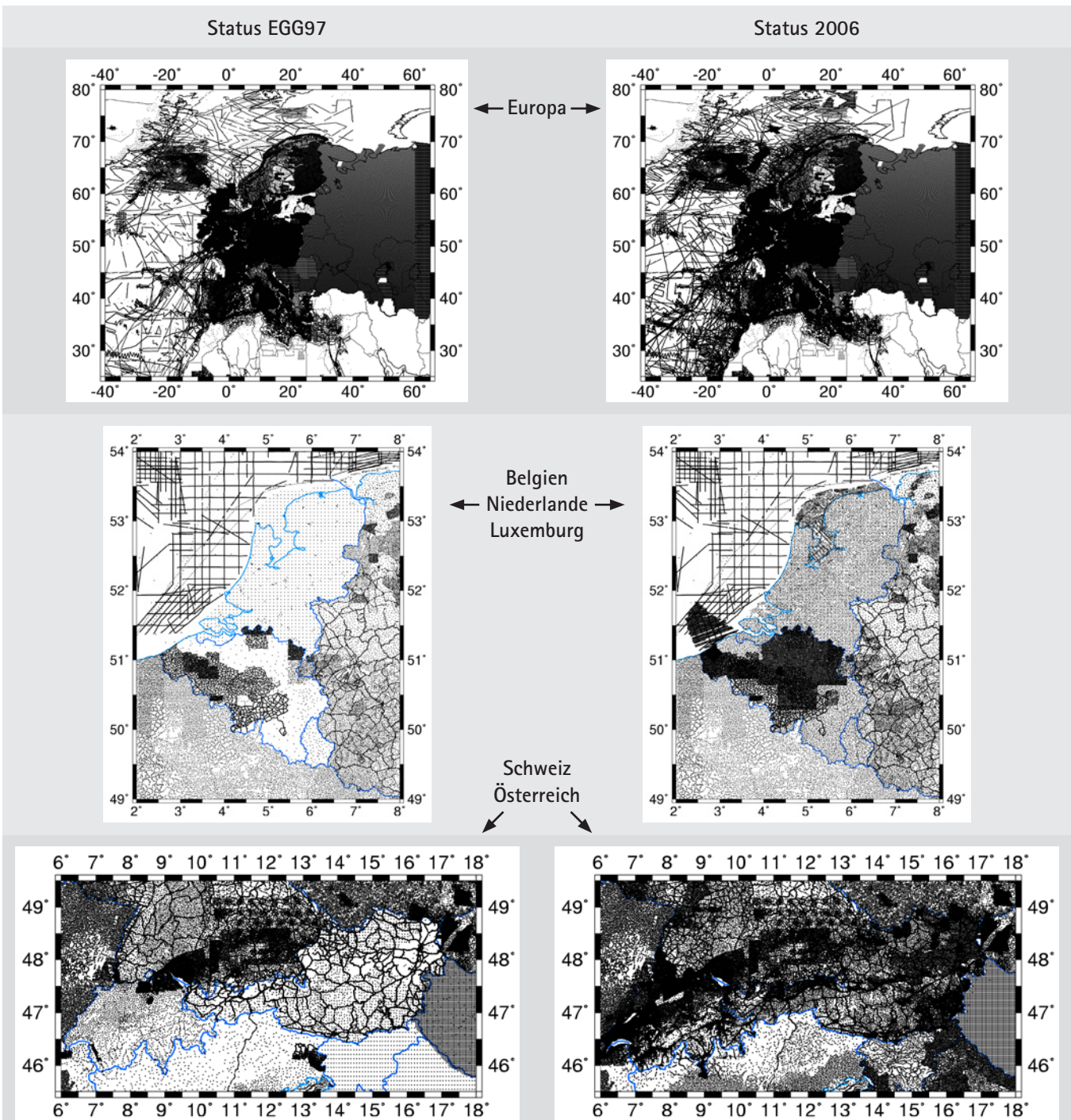
Abb. 1: Terrestrische Schweredaten für das gesamte Europa (oben), Belgien/Niederlande/Luxemburg (Mitte) und Schweiz/Österreich (unten). Im linken Teil ist jeweils der Status für das EGG97 und im rechten Teil der derzeitige Status 2006 dargestellt.
