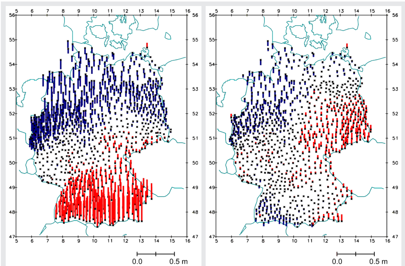
Abb. 5: Vergleich der gravimetrischen Quasigeoidlösungen EGG97 (links) und EGG06/GRACE (rechts) mit GPS- und Nivellementsdaten in Deutschland (Datensatz des BKG, s. Liebsch et al. 2006).
